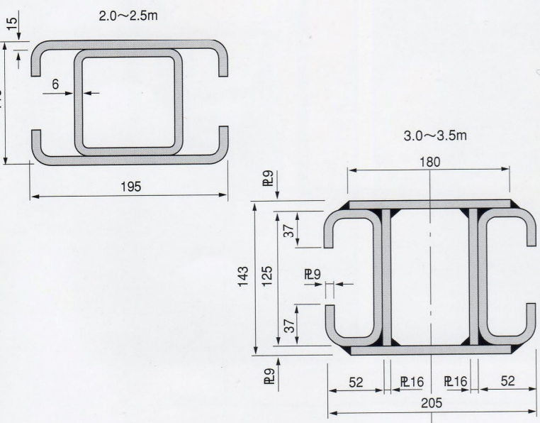
レール断面
