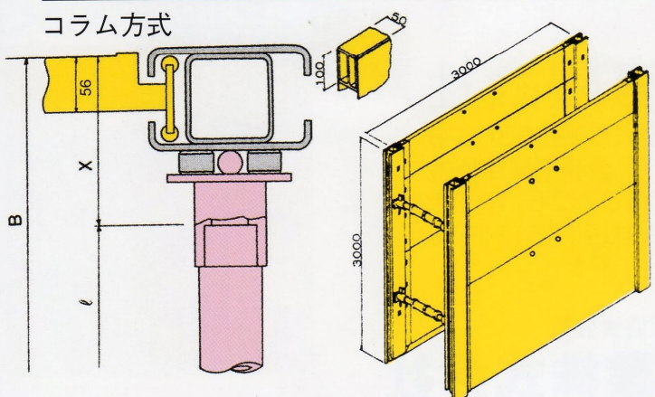
レール断面
